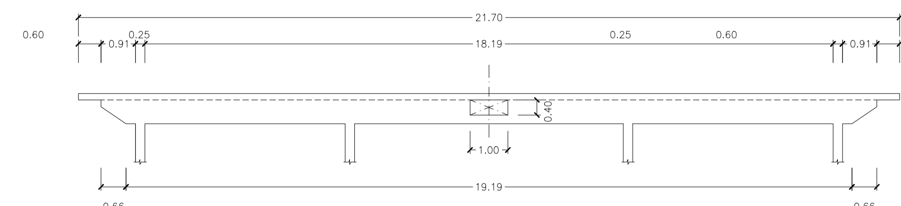
PLANTA TIPO ESQUEMA GENERAL DE 1 LINEA DE APOYO ESCALA 1:100
