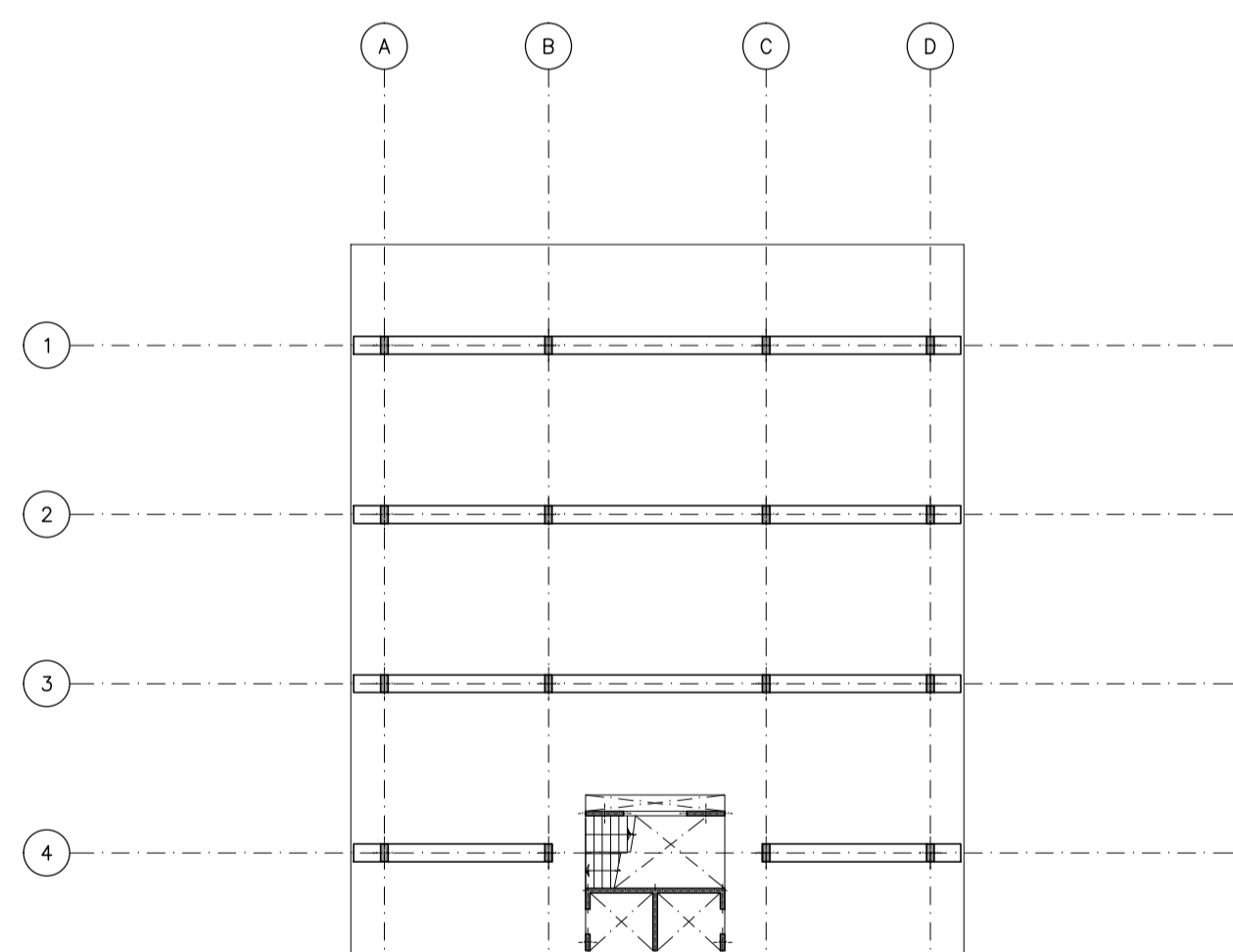
PLANTA ESQUEMÁTICA SOBRE PLANTA TIPO ESCALA 1:250
