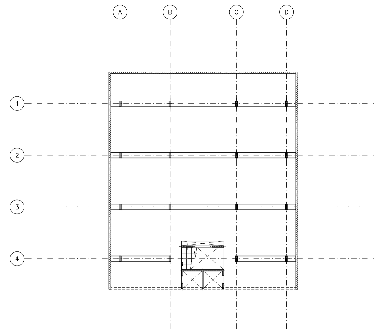
PLANTA ESQUEMÁTICA SOBRE 2º SUBSUELO ESCALA 1:250
