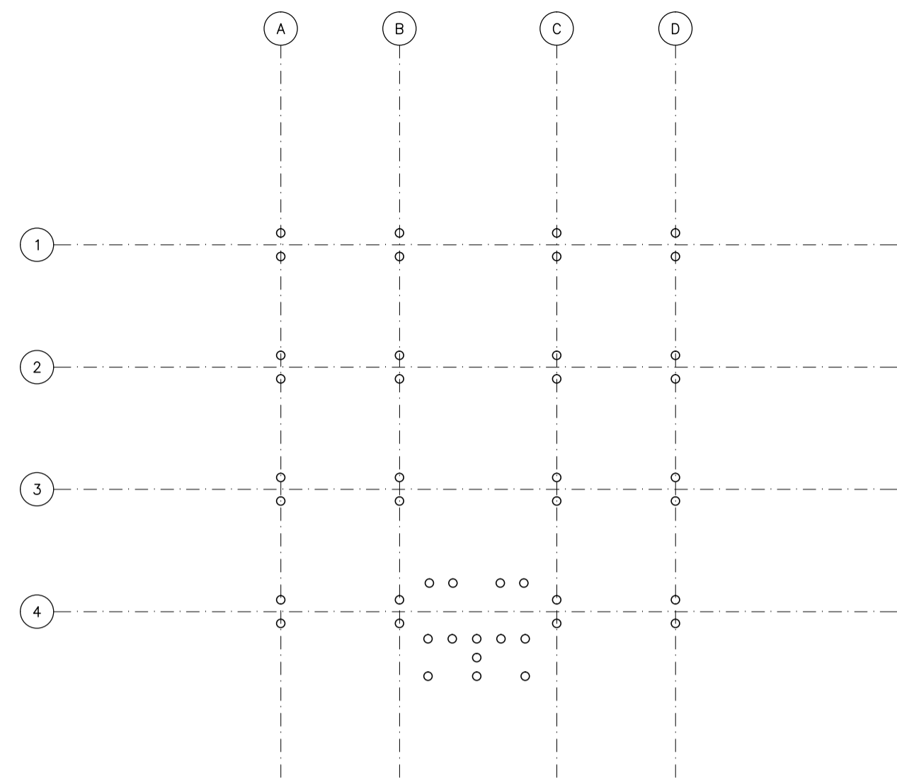
PLANTA ESQUEMÁTICA DE FUNDACIONES ESCALA 1:250
