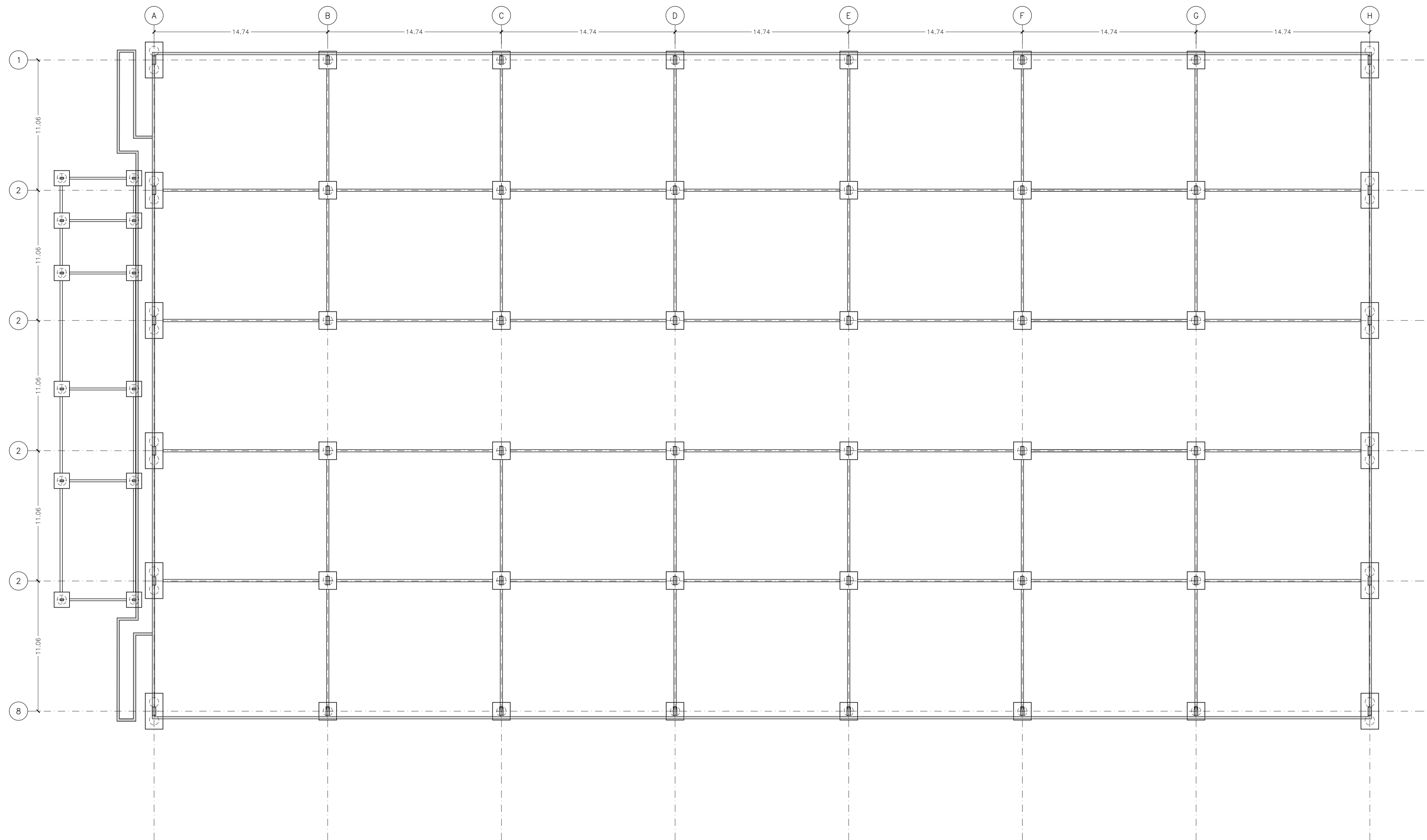
PLANTA ESQUEMÁTICA NIVEL 000 (VARIANTE CABEZALES Y PILOTES) - ESC 1:200
