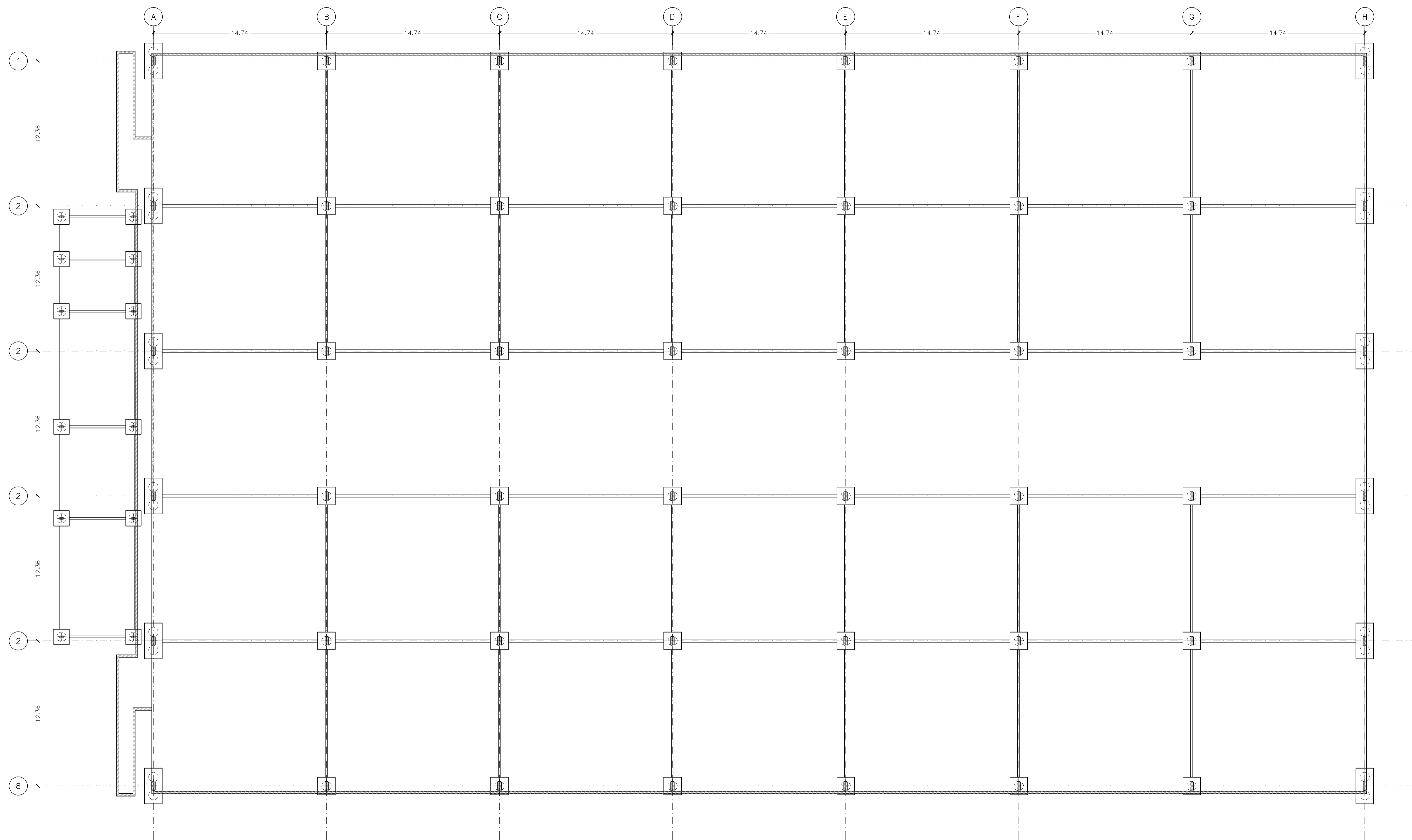
PLANTA ESQUEMÁTICA NIVEL 000 (VARIANTE CABEZALES Y PILOTES) - ESC 1:200
