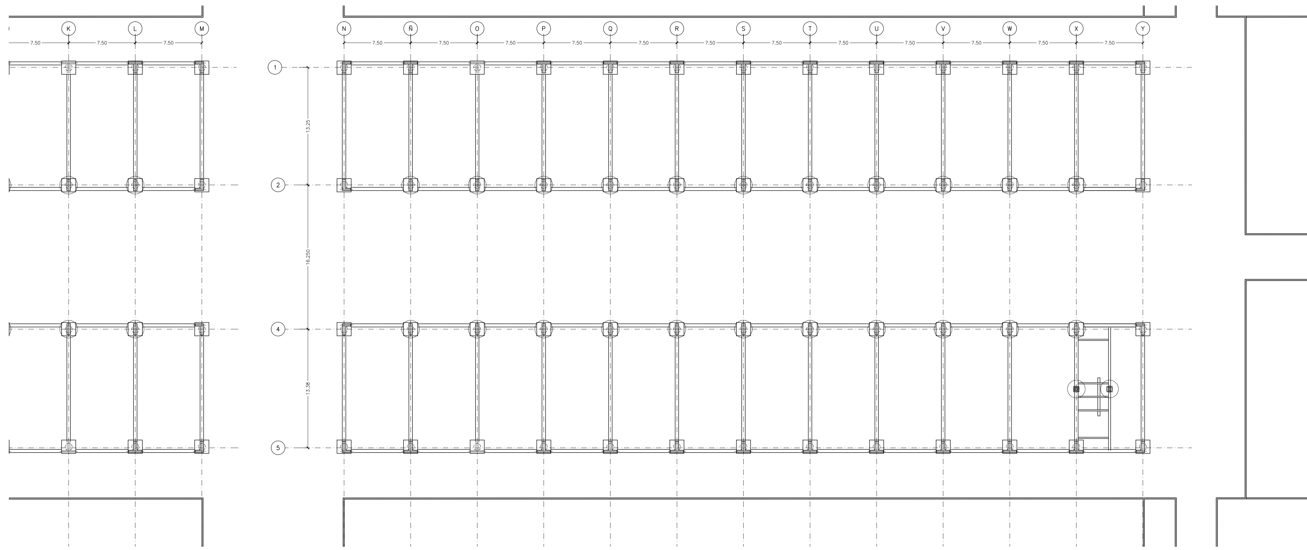
PLANTA ESQUEMATICA NIVEL 000 (VARIANTE PILOTES Y CABEZALES) - ZONA B - ESC 1:250
