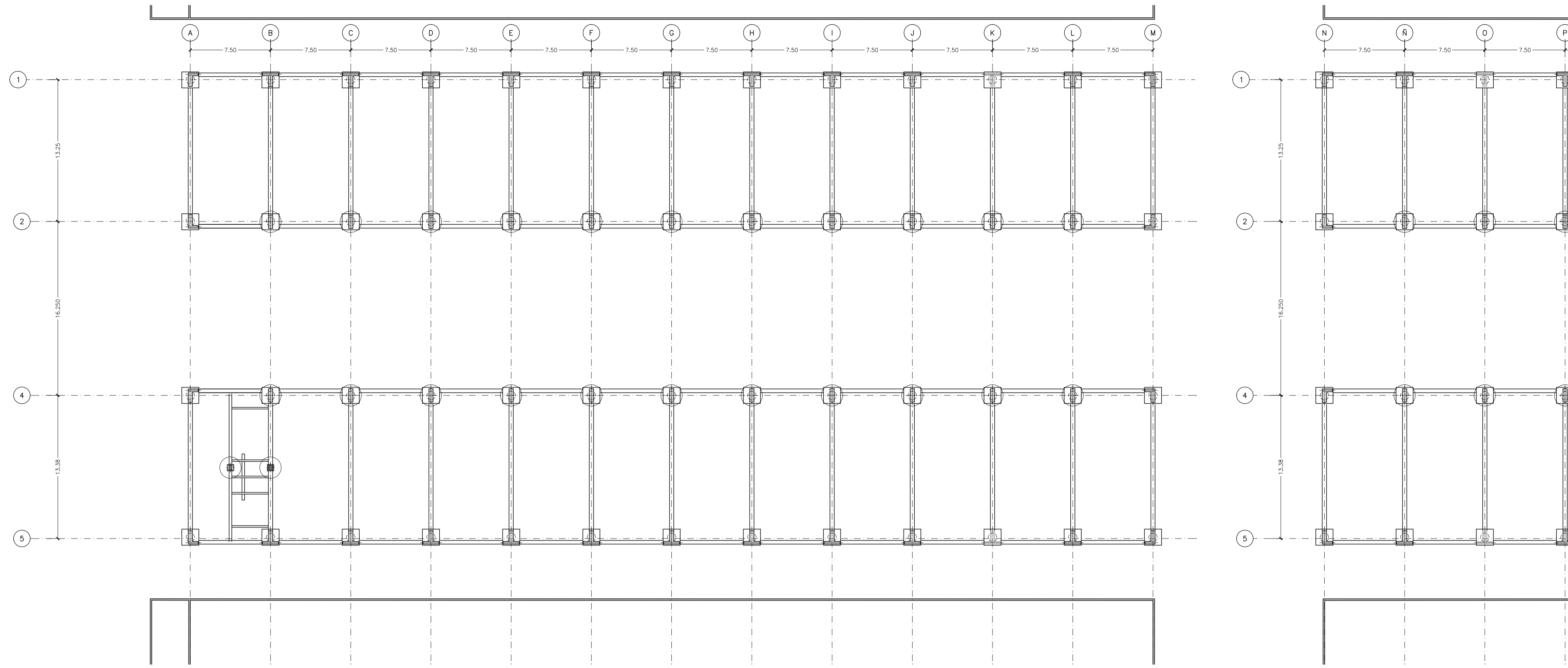
PLANTA ESQUEMATICA NIVEL 000 (VARIANTE PILOTES Y CABEZALES) - ZONA A - ESC 1:250
