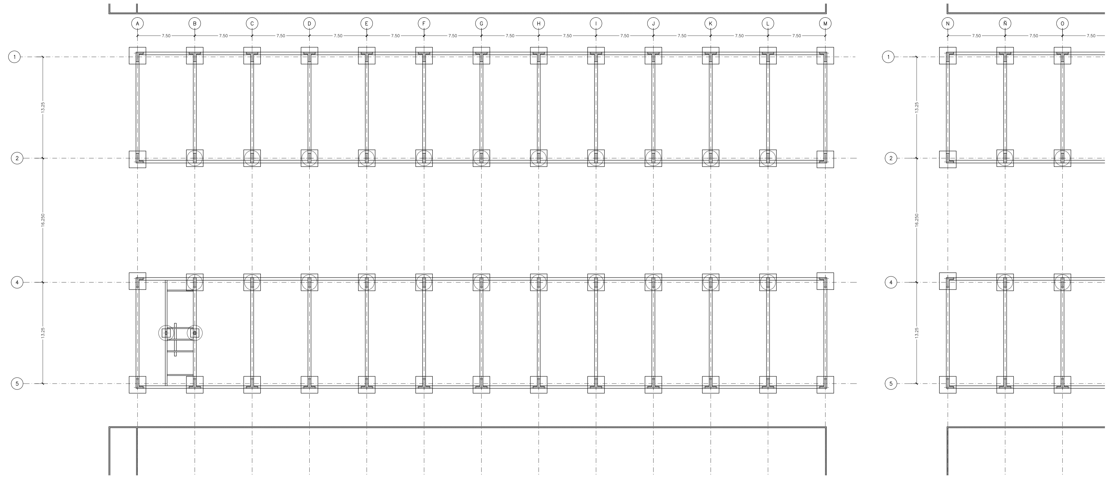
PLANTA ESQUEMATICA NIVEL 000 (VARIANTE FUNDACIÓN DIRECTA) - ZONA A - ESC 1:250
