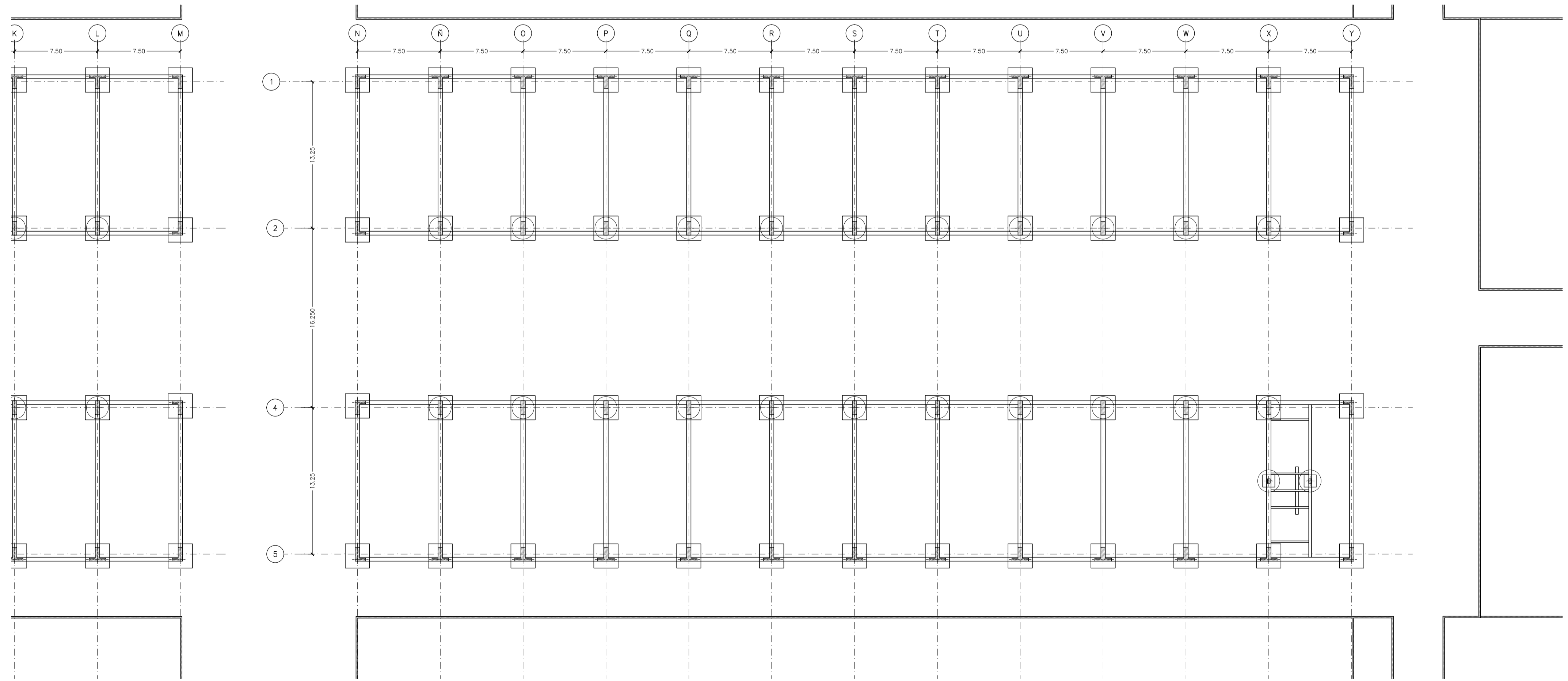
PLANTA ESQUEMATICA NIVEL 000 (VARIANTE FUNDACIÓN DIRECTA) - ZONA B - ESC 1:250
