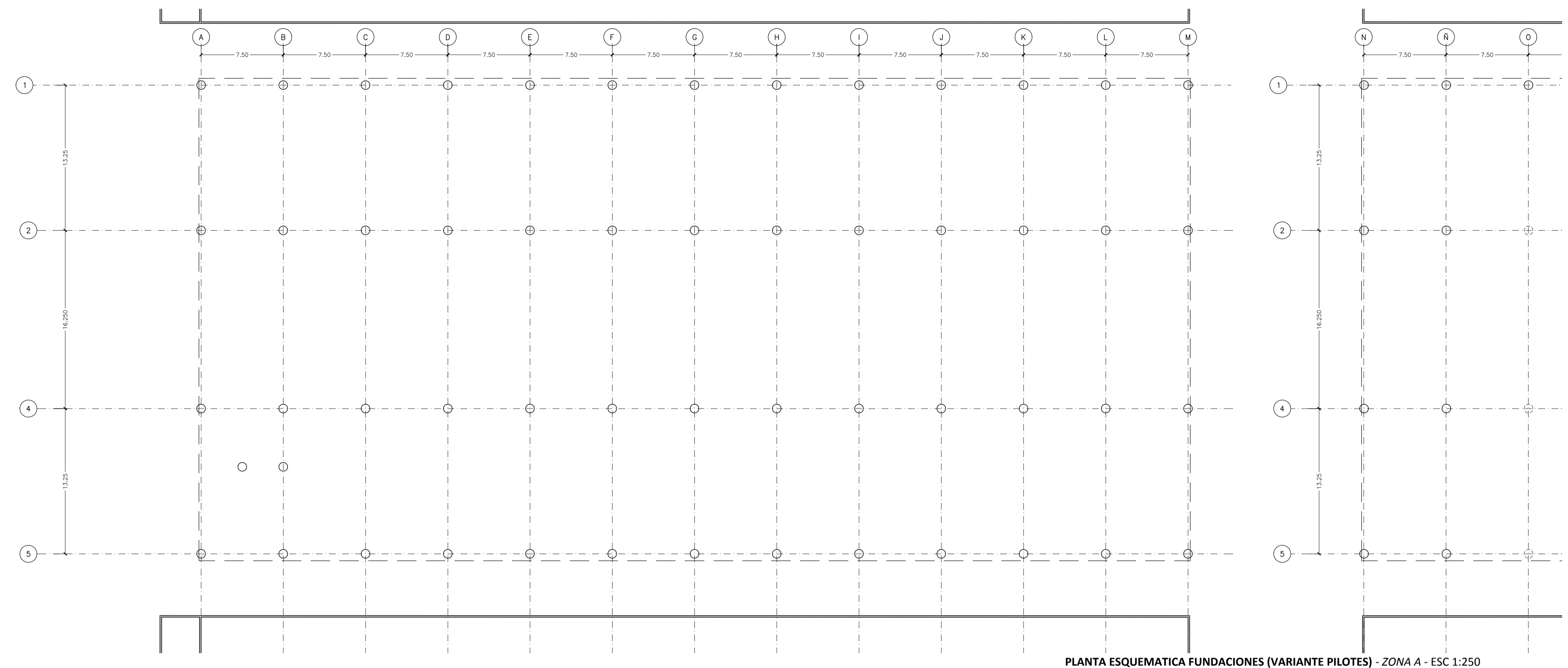
PLANTA ESQUEMATICA FUNDACIONES (VARIANTE PILOTES) - ZONA A - ESC 1:250
