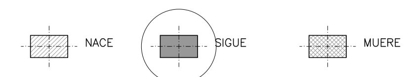
PLANTA ESQUEMATICA NIVEL 000 (VARIANTE PILOTES Y CABEZALES) - ESC 1:200
